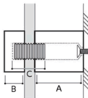
断面図 2
