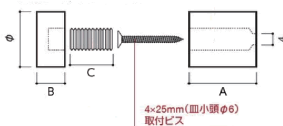
断面図 1
